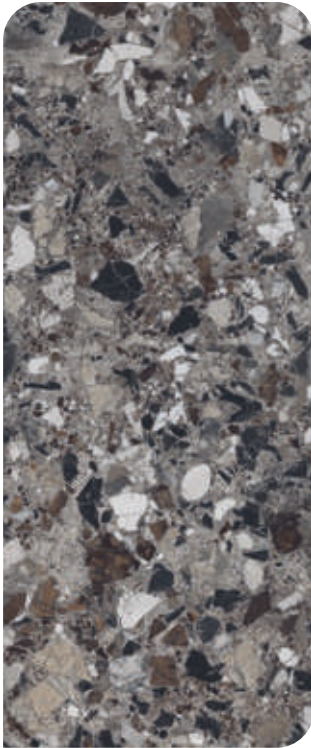
Ossidiana
