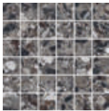
Ossidiana
