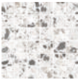
Aulite
